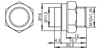
Dimensiones del racor engrampado M12x1'25
