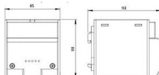
Dimensiones modelo CSL 028
